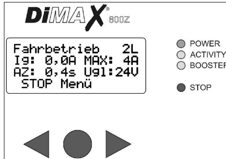
Abbildung 5: Display im Fahrbetrieb
