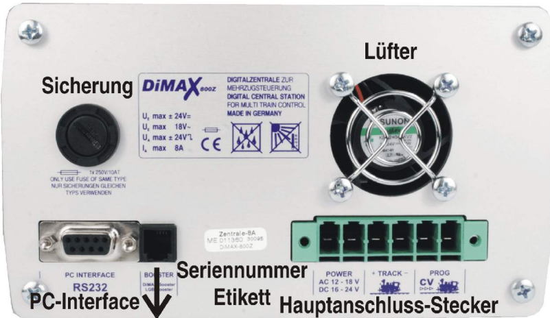
Abbildung 2: Die Rückansicht der DiMAX
