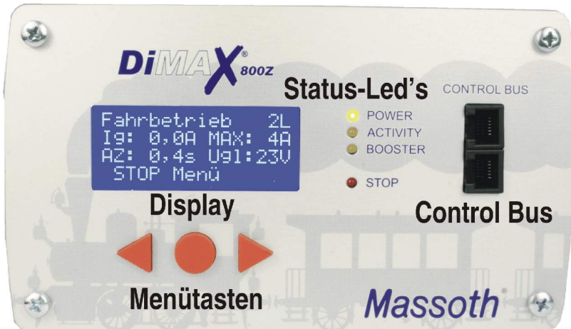
Abbildung 1: Die Frontansicht der DiMAX
