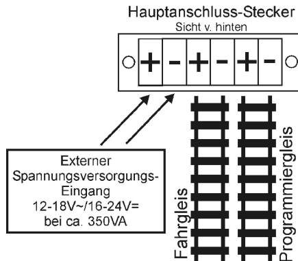
Abbildung 3: Steckeranschluss
